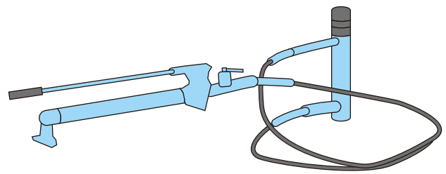
■複動式ジャッキと手動ポンプ
